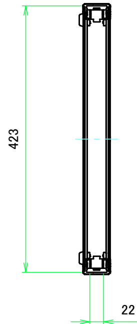
A-A (1:6)
