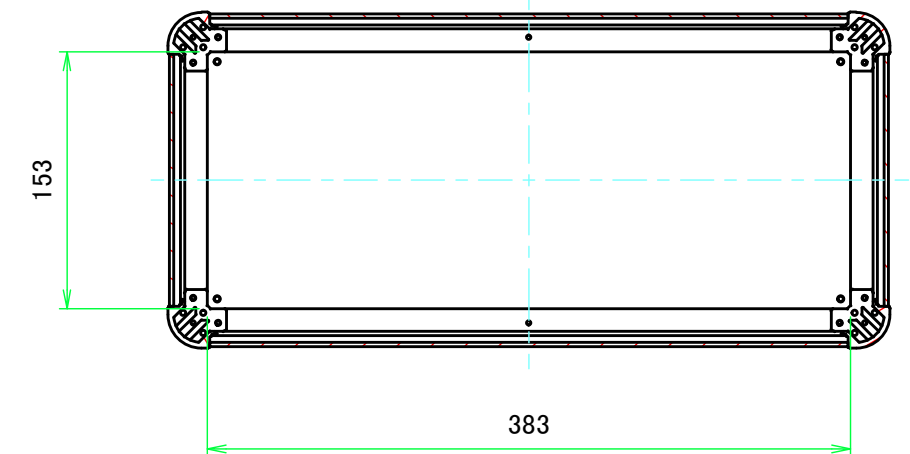
C-C (1 : 4.5)
