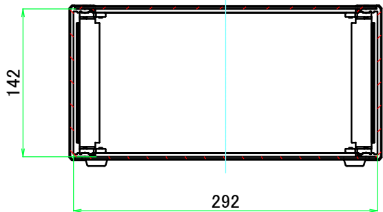
B-B ( 1 : 5 )
