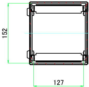
A-A ( 1 : 5 )
