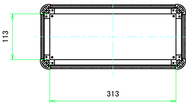
C-C ( 1 : 5.5 )
