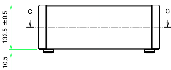
B-B ( 1 : 5.5 )
