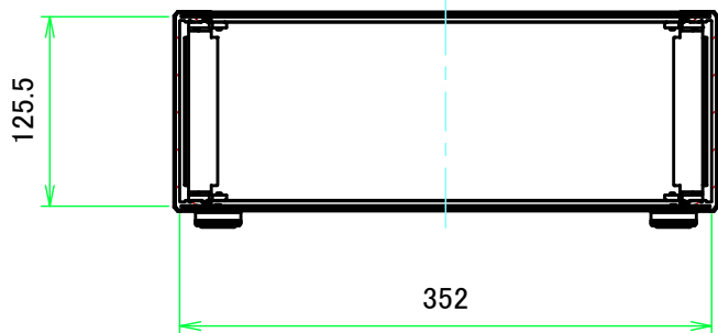
B-B ( 1 : 5.5 )
