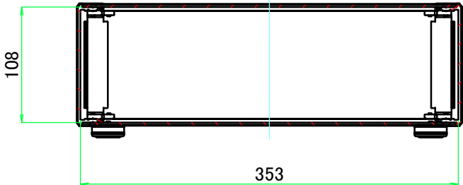
A-A (1:5)
