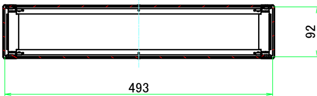
C-C ( 1 : 7 )
