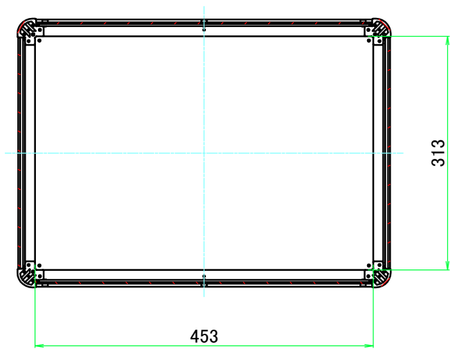
B-B ( 1 : 7 )
