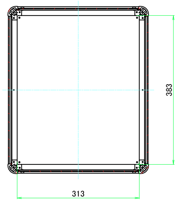
B-B ( 1 : 6 )
