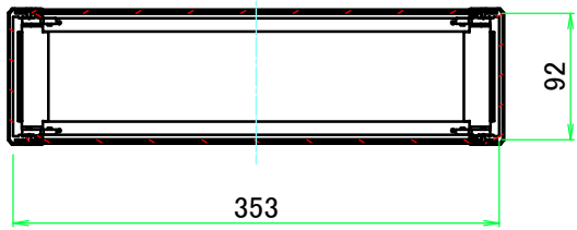
C-C ( 1 : 6 )
