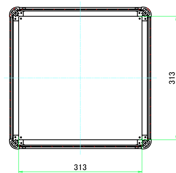
B-B ( 1 : 6 )
