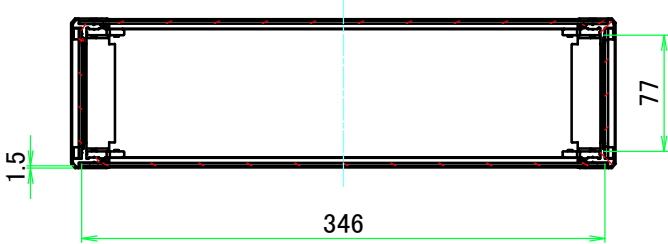
A-A (1:5)
