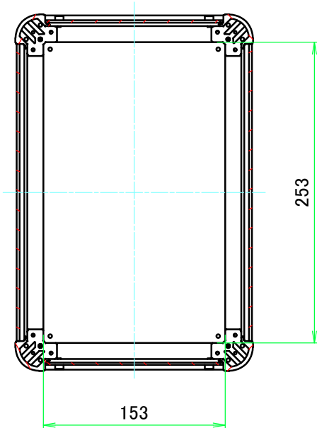
B-B ( 1 : 4.5 )
