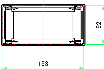
C-C ( 1 : 4.5 )
