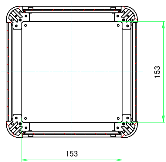
B-B ( 1 : 3.5 )
