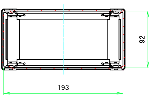
C-C ( 1 : 3.5 )
