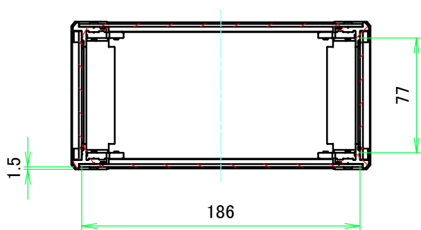
A-A ( 1 : 3.5 )
