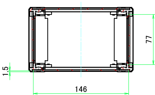
A-A ( 1 : 3.5 )
