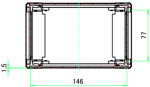
A-A (1:3)
