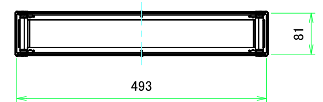
C-C ( 1 : 7.5 )
