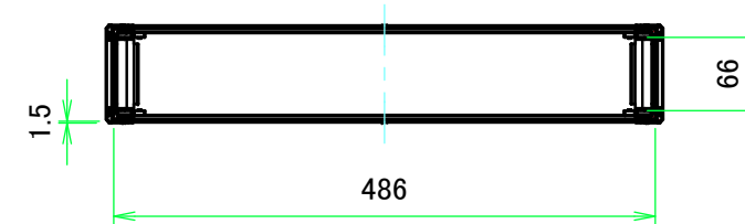
A-A ( 1 : 7.5 )
