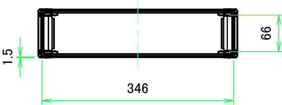
A-A ( 1 : 7 )
