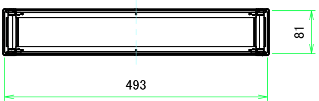
C-C ( 1 : 7 )
