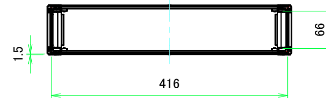
A-A ( 1 : 6.5 )
