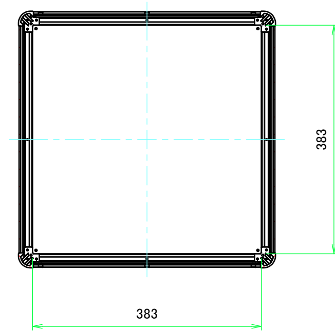
B-B ( 1 : 6.5 )
