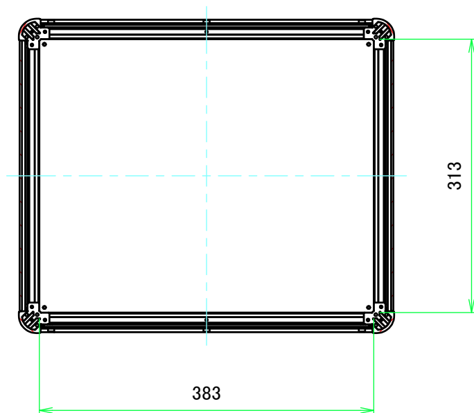
B-B ( 1 : 6 )
