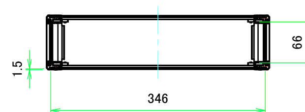
A-A ( 1 : 6 )
