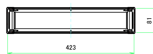
C-C ( 1 : 6 )
