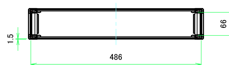
A-A ( 1 : 6.5 )
