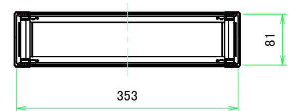
C-C ( 1 : 6 )
