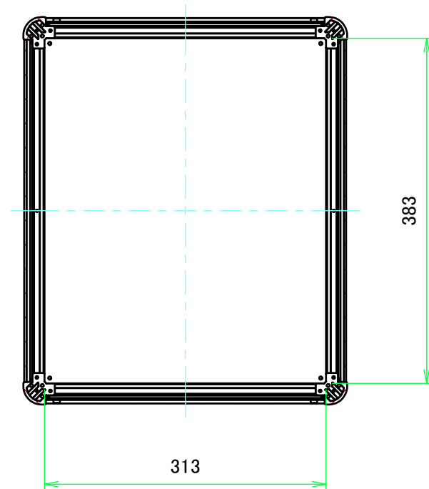
B-B ( 1 : 6 )
