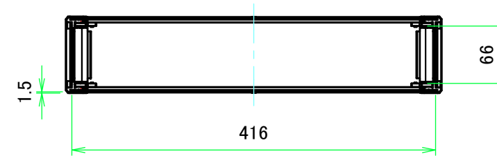
A-A ( 1 : 6 )
