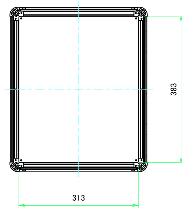
B-B ( 1 : 6 )
