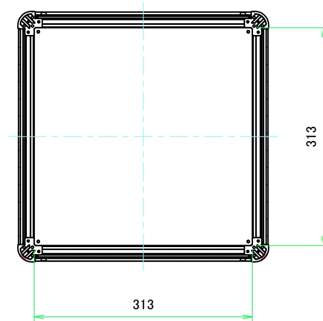
B-B ( 1 : 5.5 )
