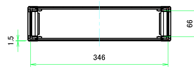
A-A ( 1 : 5.5 )
