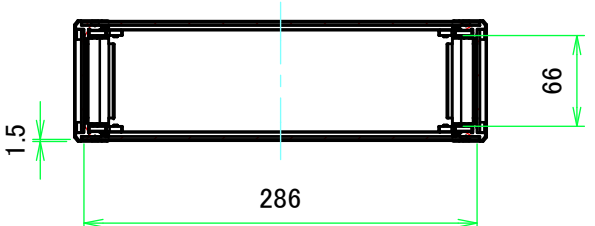
A-A ( 1 : 5.5 )
