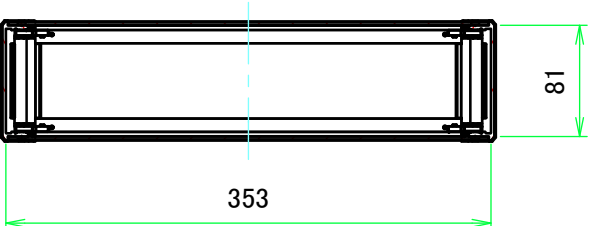
C-C ( 1 : 5.5 )
