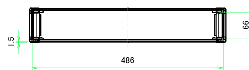
A-A ( 1 : 6 )
