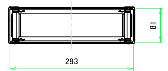
C-C ( 1 : 5.5 )
