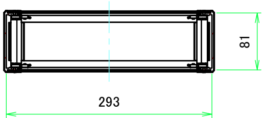
C-C ( 1 : 5.5 )
