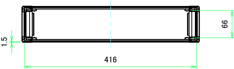
A-A ( 1 : 5.5 )
