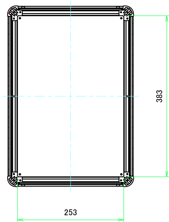
B-B ( 1 : 5.5 )
