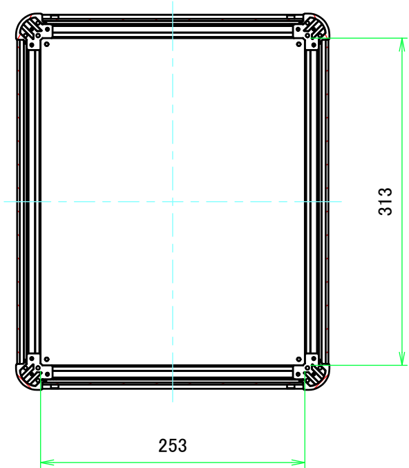
B-B ( 1 : 5 )
