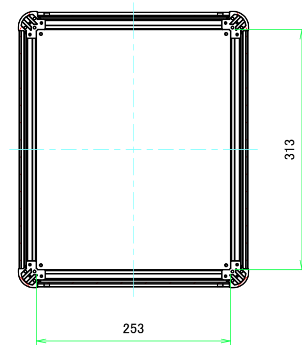
B-B ( 1 : 5 )
