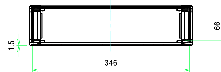
A-A ( 1 : 5 )
