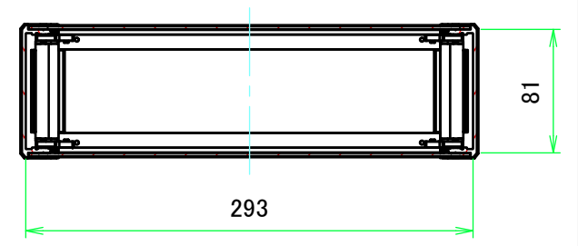
C-C ( 1 : 4.5 )
