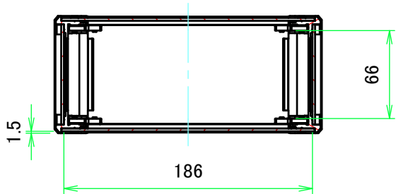
A-A ( 1 : 4 )
