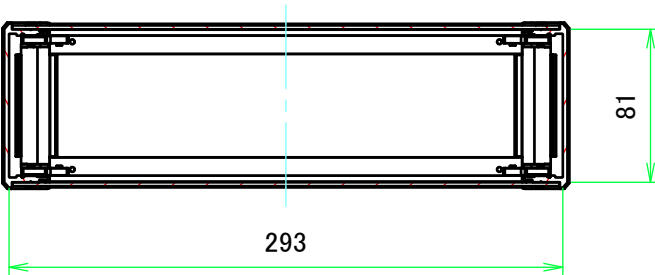
C-C ( 1 : 4 )
