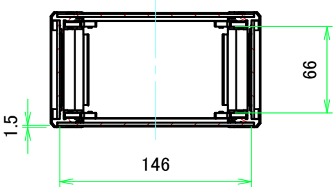
A-A ( 1 : 4 )
