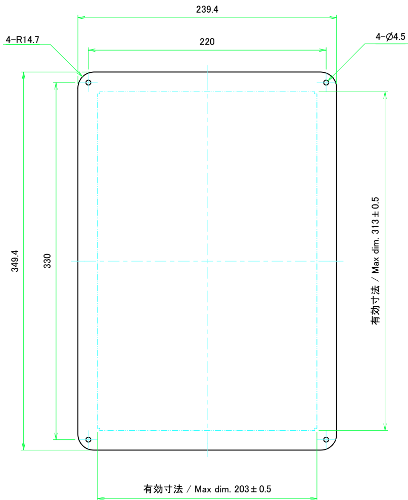
保護シート側 Surface protective film side
