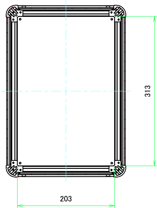
B-B ( 1 : 4.5 )
