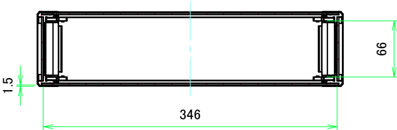
A-A ( 1 : 4.5 )
