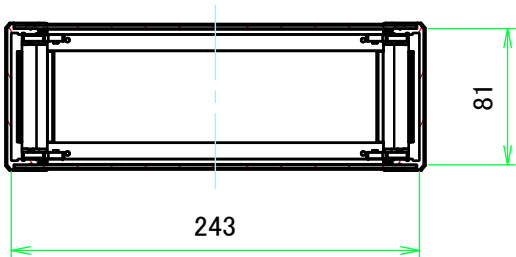
C-C ( 1 : 4.5 )
