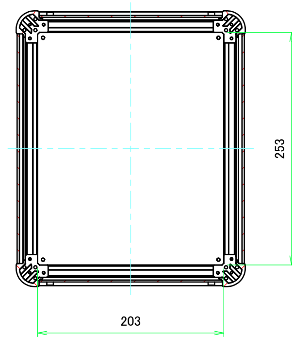
B-B ( 1 : 4 )
