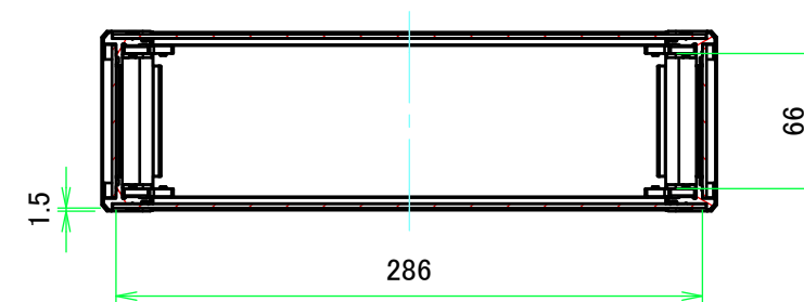
A-A ( 1 : 4 )
