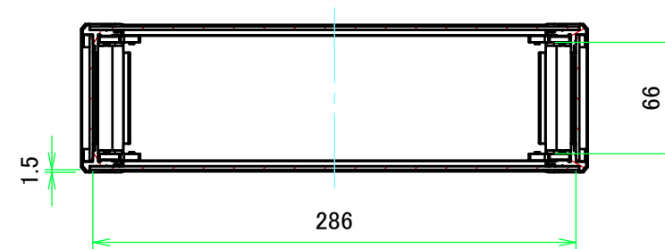
A-A ( 1 : 4 )
