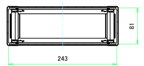
C-C ( 1 : 4 )
