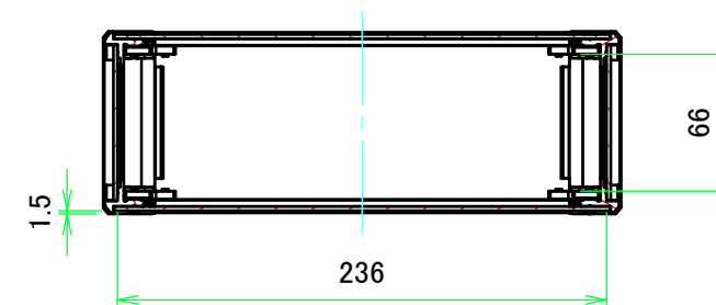
A-A (1:4)
