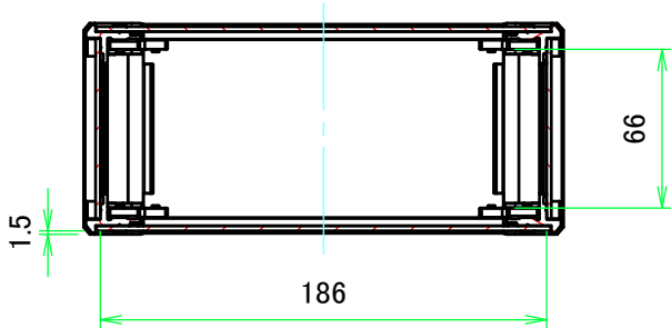
A-A ( 1 : 3.5 )
