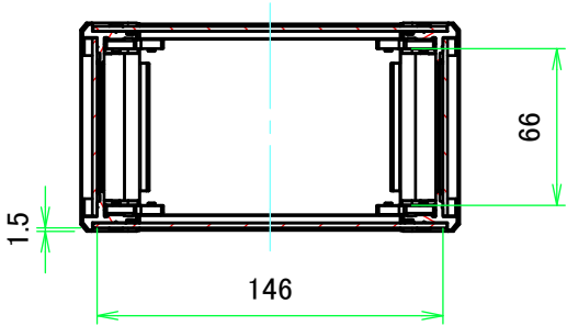
A-A ( 1 : 3.5 )
