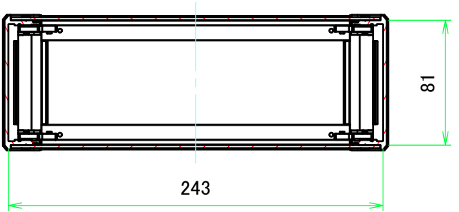
C-C ( 1 : 3.5 )
