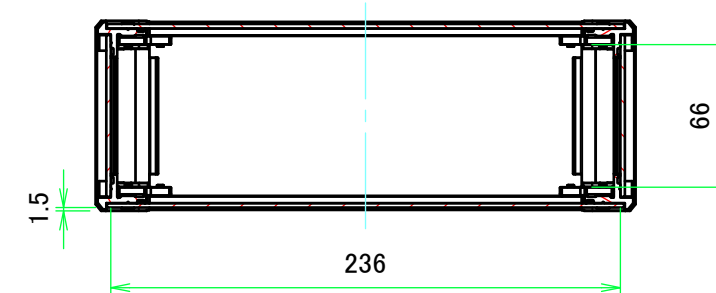
A-A ( 1 : 3.5 )
