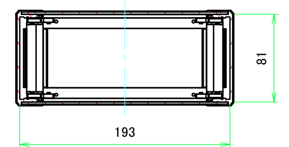
C-C ( 1 : 3.5 )
