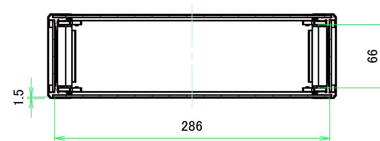
A-A (1:4)
