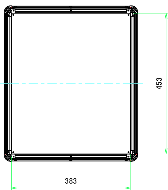
B-B ( 1:7 )
