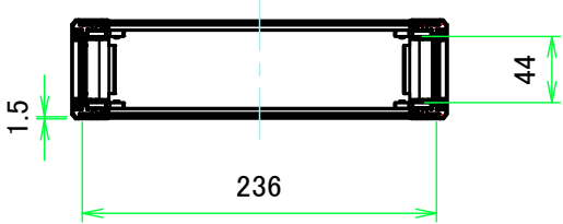
A-A ( 1:5.5 )
