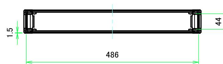
A-A ( 1:6.5 )
