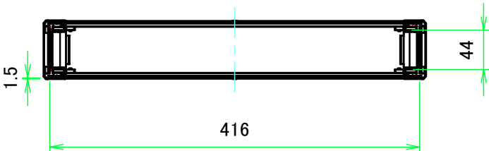
A-A ( 1:6 )
