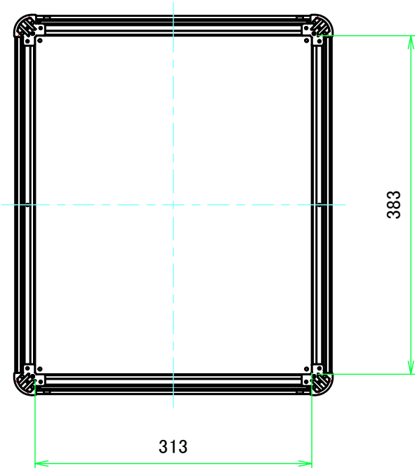
B-B ( 1:6 )
