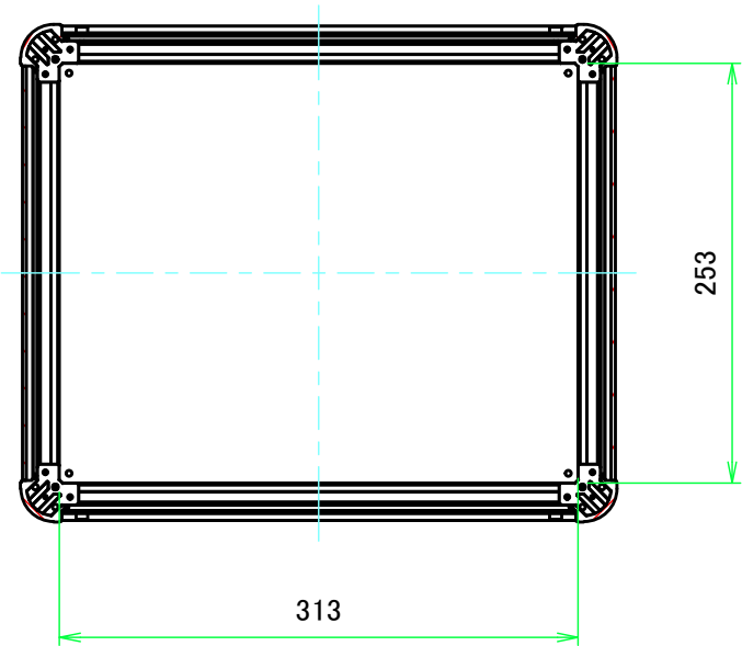
B-B ( 1:5 )
