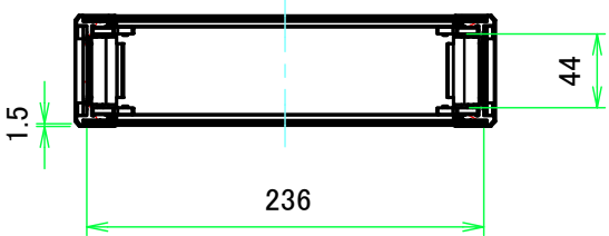
A-A ( 1:5 )
