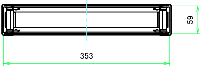
C-C ( 1:5 )
