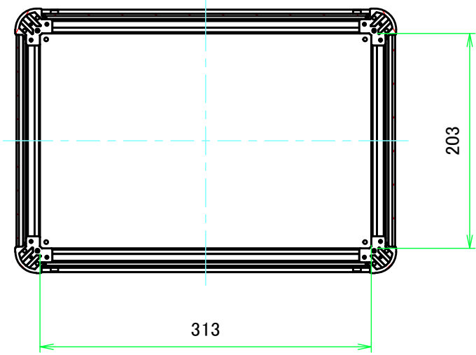
B-B ( 1:5 )
