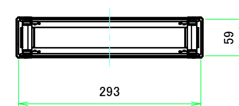
C-C ( 1:6 )
