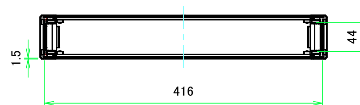
A-A ( 1:5.5 )
