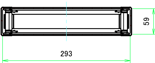
C-C ( 1:5 )
