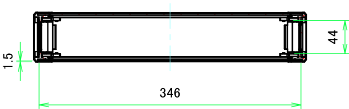
A-A ( 1:5 )
