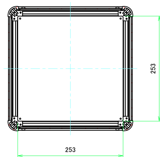
B-B ( 1:4.5 )
