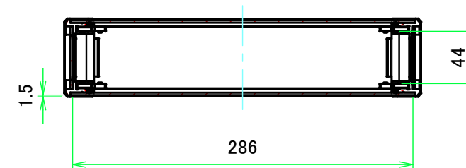
A-A ( 1:4.5 )
